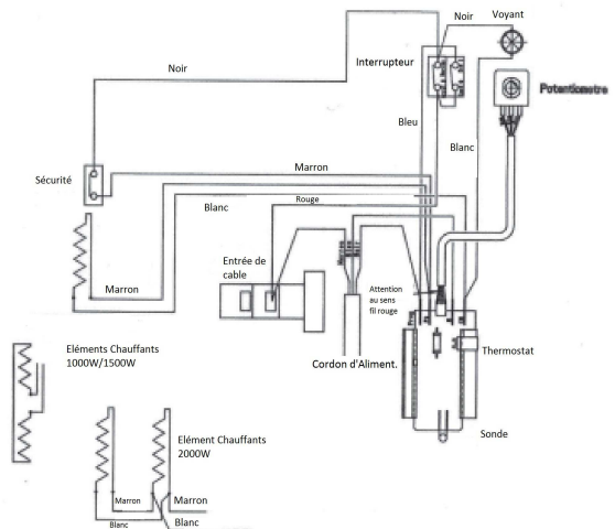
Schéma Electrique indice 03-05
