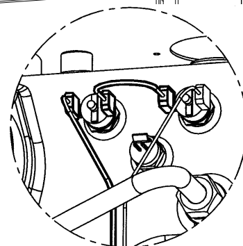
Câblage à réaliser pour un fonctionnement basse température avec limitation haute à 60°C.
