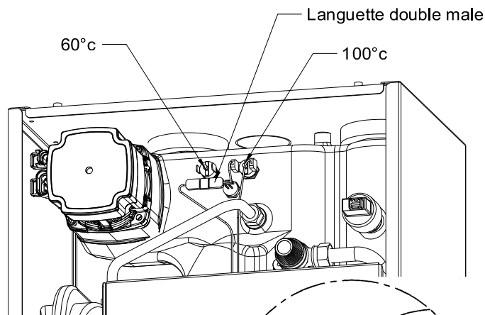
Aquastats de sécurité à réarmement manuel Câblage d'usine pour un fonctionnement haute température avec limitation haute à 100°C
